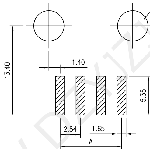
P.C.B LAYOUT
